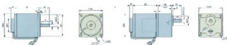
( )内值为5GN3-5GN20之尺寸 * 表示5GN20-5GN180之尺寸 方键: 4X4X25
