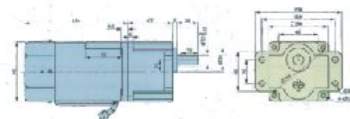
5GU口 方键：5X5X25
