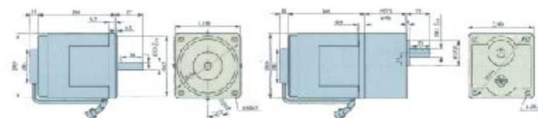
( )内值为5GN3-5GN20之尺寸 * 表示5GN20-5GN180之尺寸 方型: 4X4X25
