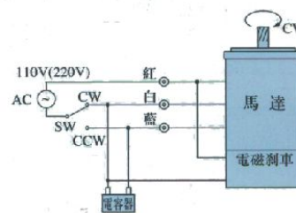
■单相刹车马达接线图
